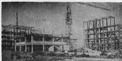
БАЗА ХЕМИЈА — НАЈЗНАЧАЈНИЈА ИНВЕСТИЦИЈА У ИСТОРИЈИ „ПРВЕ ИСКРЕ“. Завршетак објеката ТДИ и ЛАП очекује се до краја ове године. Пробна производња почиње наредне године да би се уложили сложени технолошки поступци. Ови објекти ће омогућити да „Прва искра“ постане изразити извозник.
